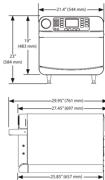
Encore 2 Oven Dimensions
